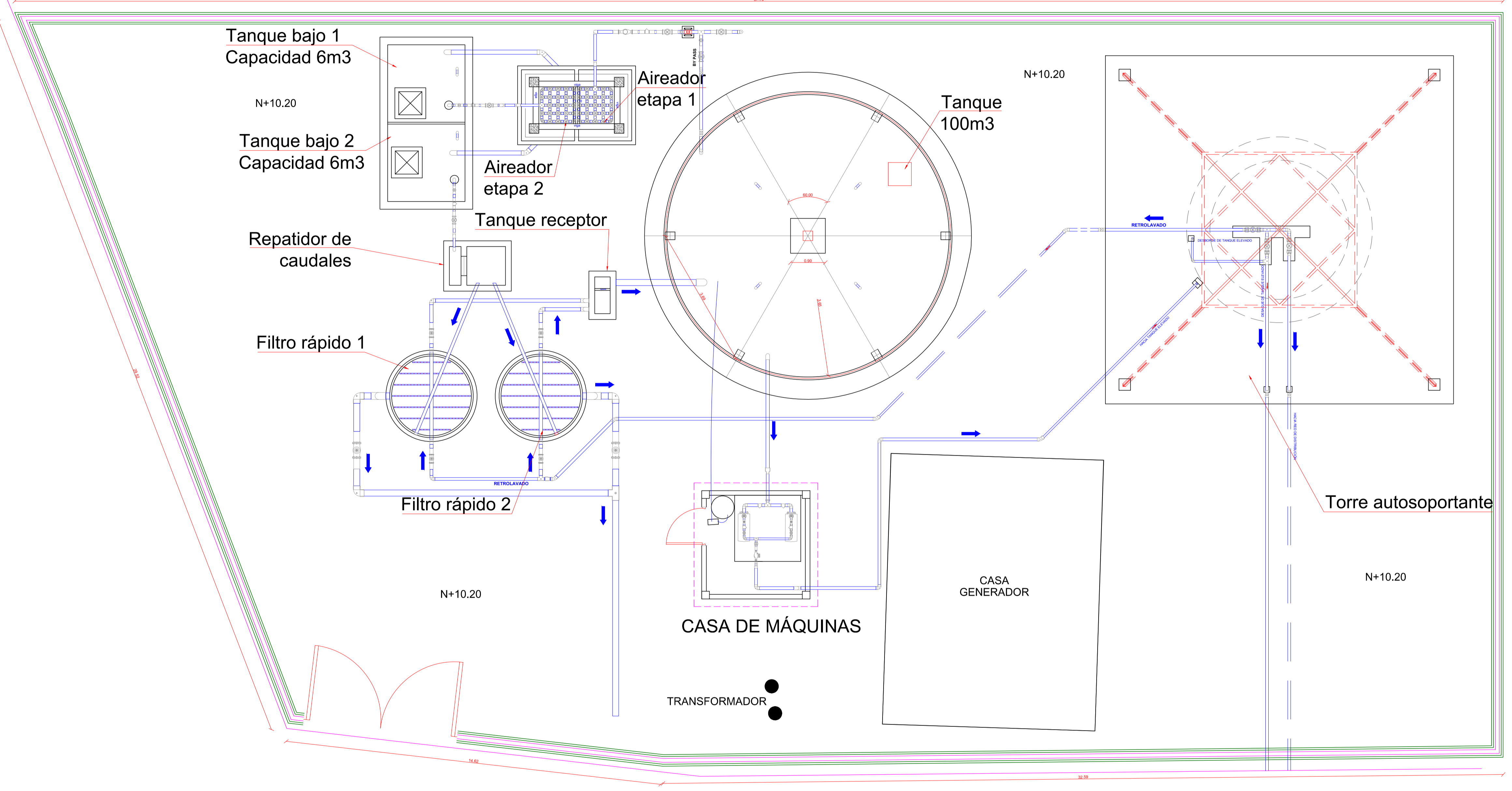
IMPLANTACIÓN PLANTA DE POTABILIZACIÓN DE AGUA Escala: _____ S/E
